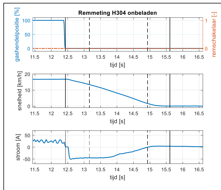
Figuur 13: Remmetingen H304; onbeladen, zonder bediening van de remhendel
