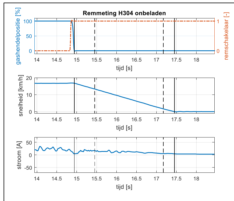
Figuur 14: Remmetingen H304; onbeladen met bekrachtiging van de remhendel
